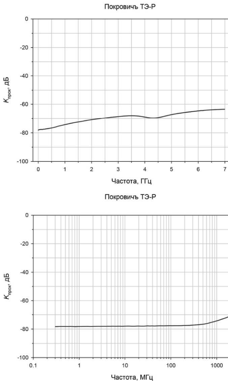
Рисунок 1 – Частотная зависимость коэффициента пропускания ЭМИ для образца ткани «Покровиць ТЭ-80»
