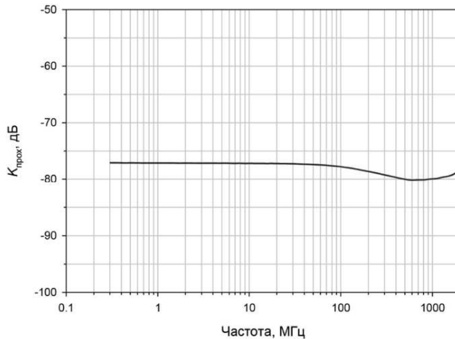
Рисунок 1 – Частотная зависимость коэффициента пропускания ЭМИ для образца ткани «Покровичь ТЭ-110»
